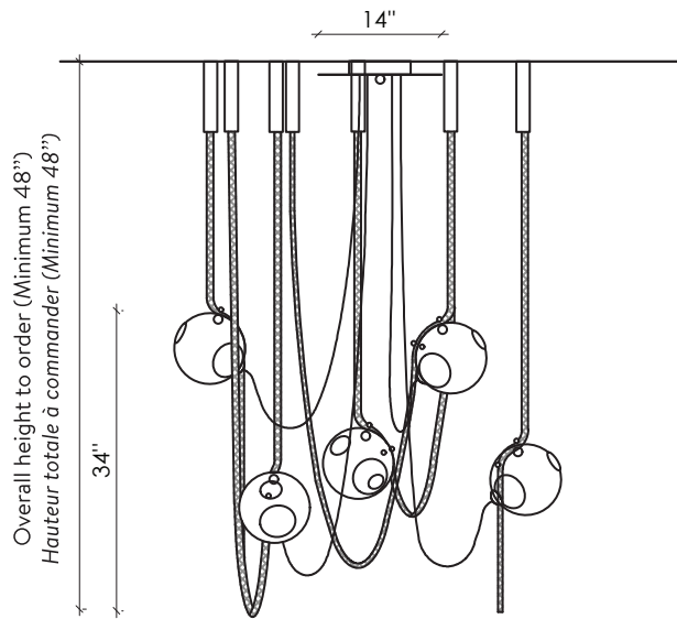
FRONT VIEW VUE DE FACE
